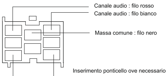
Schema montaggio ponticello ove necessario
